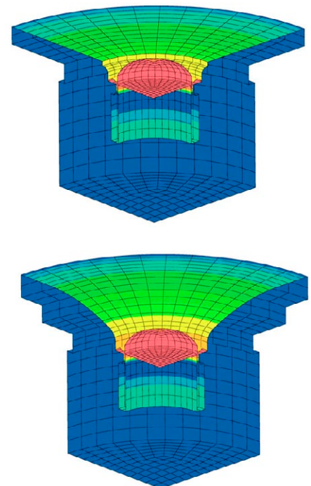
Canton optimierte das Abstrahlverhalten der Hochtonkalotte, indem eine Schallführung rund um den Dom gelegt wurde. Hierdurch konnte auch der Wirkungsgrad gesteigert werden. Oben der Tweeter aus der Vorgängerserie, unten das überarbeitete, neue Chassis
